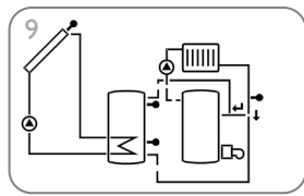
Solaranlage mit Heizkreis-Rücklaufanhebung (Seite 42)
