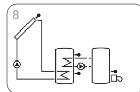
Solaranlage mit Nachheizung durch Festbrennstoffkessel (Seite 36)
