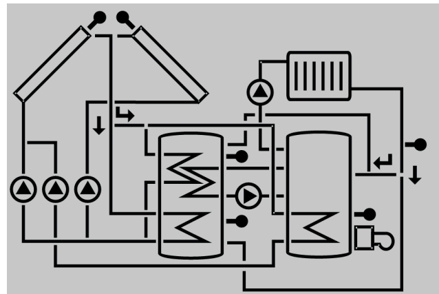
Kollektoren mit Kollektorsensor
