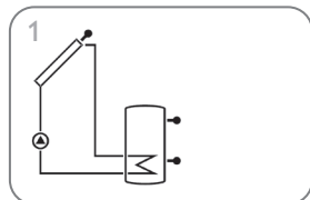
Standard-Solaranlage (Seite 10)
