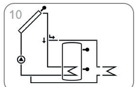
Standard-Solaranlage mit Überwärmabfuhr (Seite 45)
