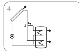
Solaranlage mit Speicherschichtbelastung (Seite 24)
