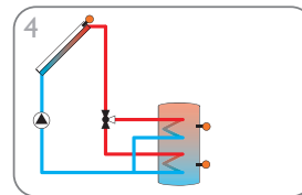
Solarsystem mit 1 Speicher und 3-Wege-Ventil zur Speicherschichtladung (Seite 13)
