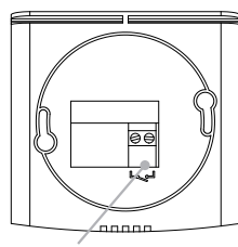
Liitäntä GSM-kytkimelle
